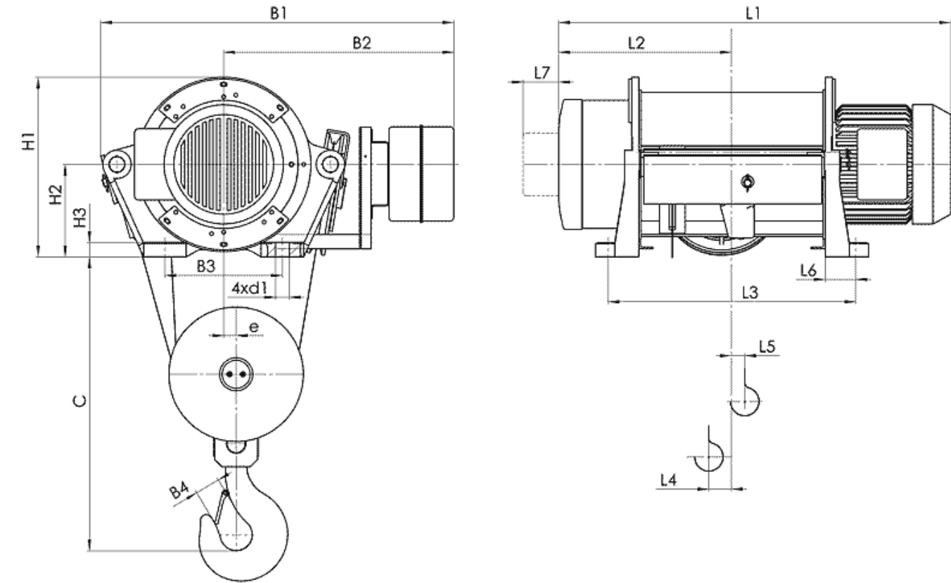
Канатный электротельфер Т35 Стационарный (подвесной) на лапах, полиспаст 4/1
