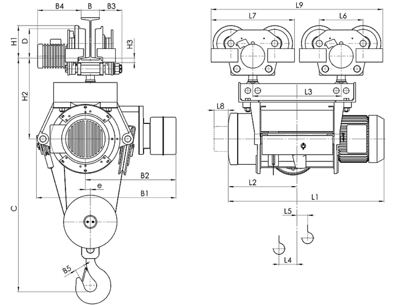
Канатный электротельфер Т39 Передвигаемый двумя тележками, полиспаст 4/1
