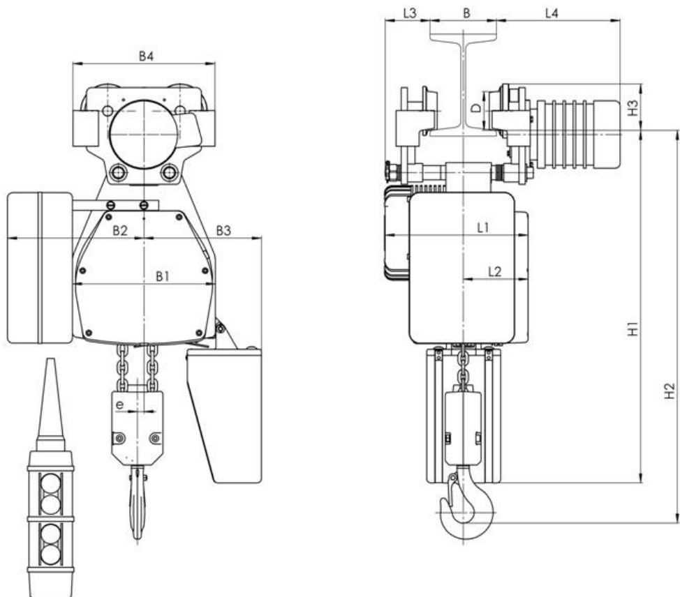
Ланцюговий електротельфер типу ВЕ, що переміщується за допомогою моторного візка
