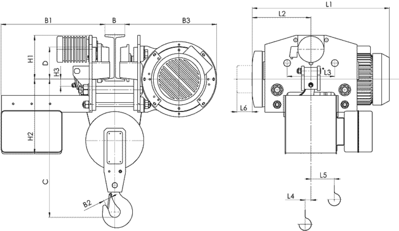
Канатный электротельфер Т45 Уменьшенная строительная высота, полиспаст 2/1
