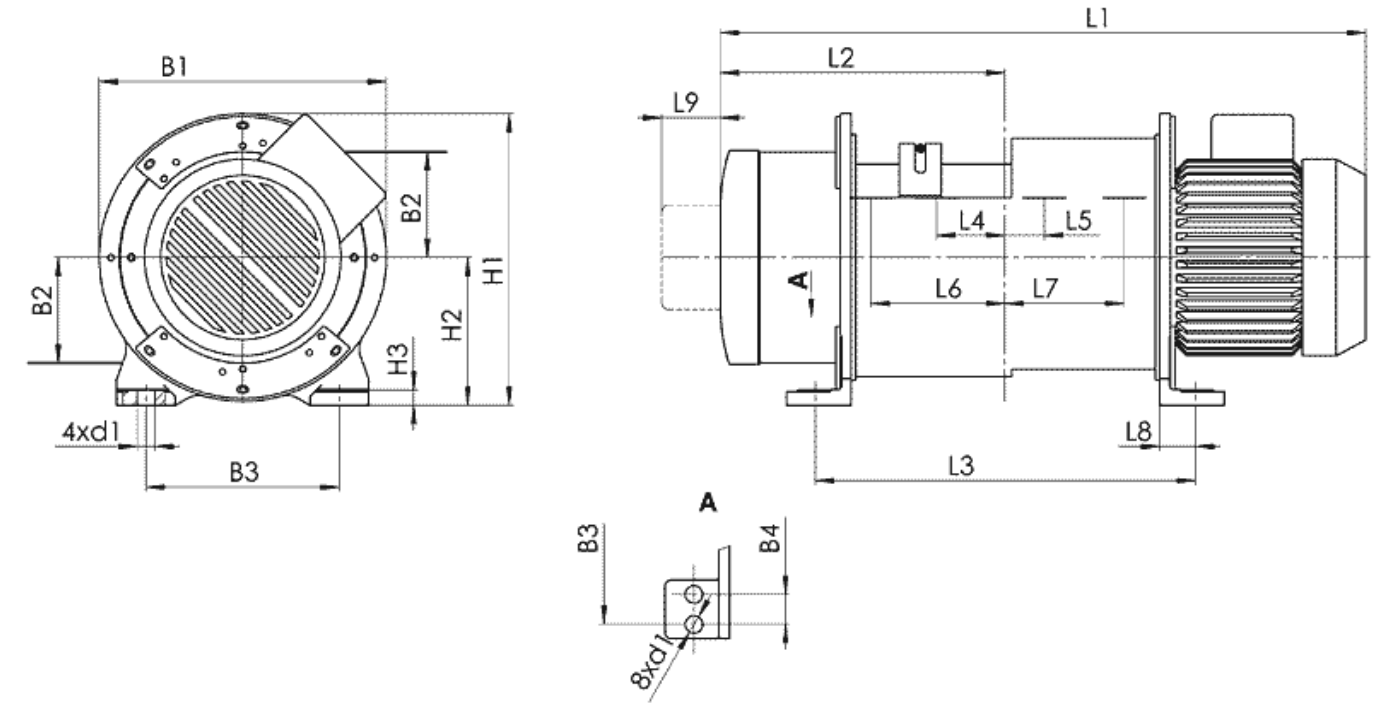
Канатный электротельфер Т52 Стационарный (подвесной) на лапах, полиспаст 2/2
