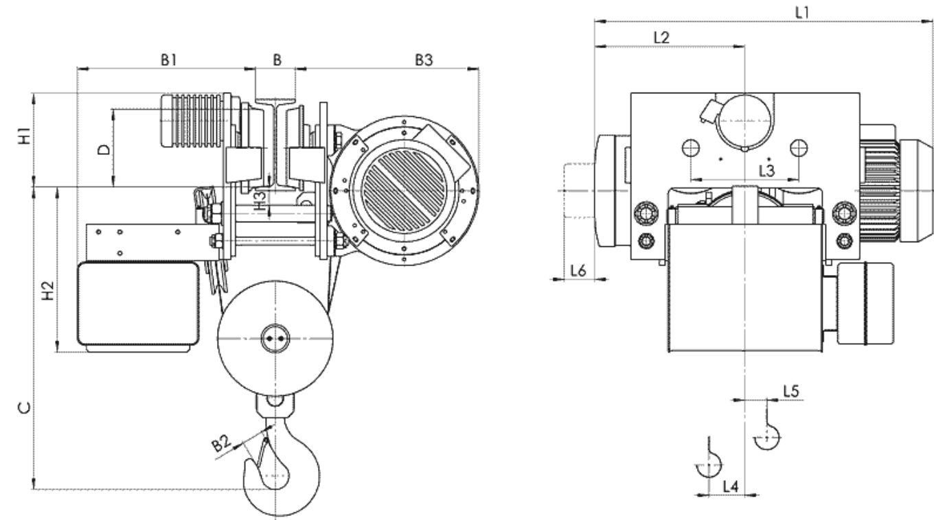
Канатный электротельфер Т78 Уменьшенная строительная высота, полиспаст 4/1
